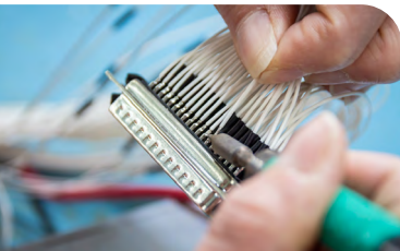
Pájení drátů ke konektoru.
